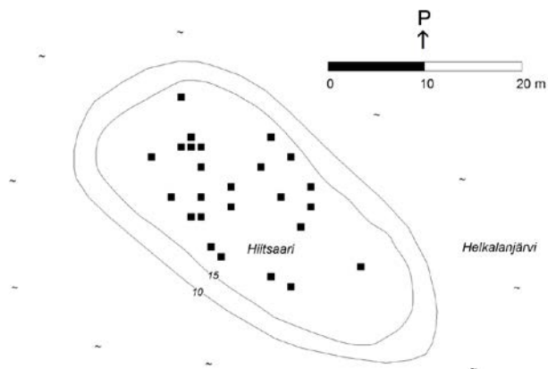
Kuva 4. Hiitsaaresta havaitut hautapainanteet ja niiden sijainti gps-laitteella mitattuna.
