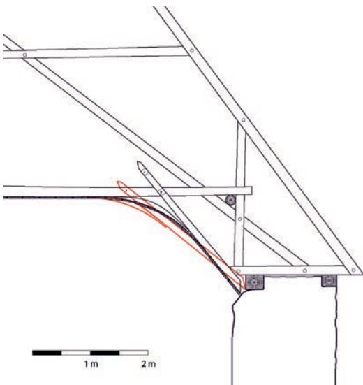
Kuva 12. Leikkauspiirustus laipion rakenteen muutoksesta. Punaisella alkuperäinen loivempi rakenne. Piirros: Laura Laine.
