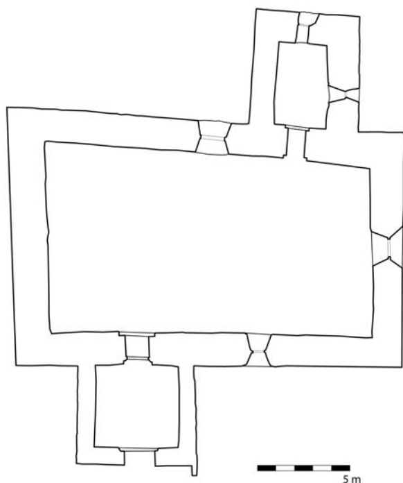
Kuva 3. Keminmaan kirkon pohjapiirros. Piirros: Laura Laine.
